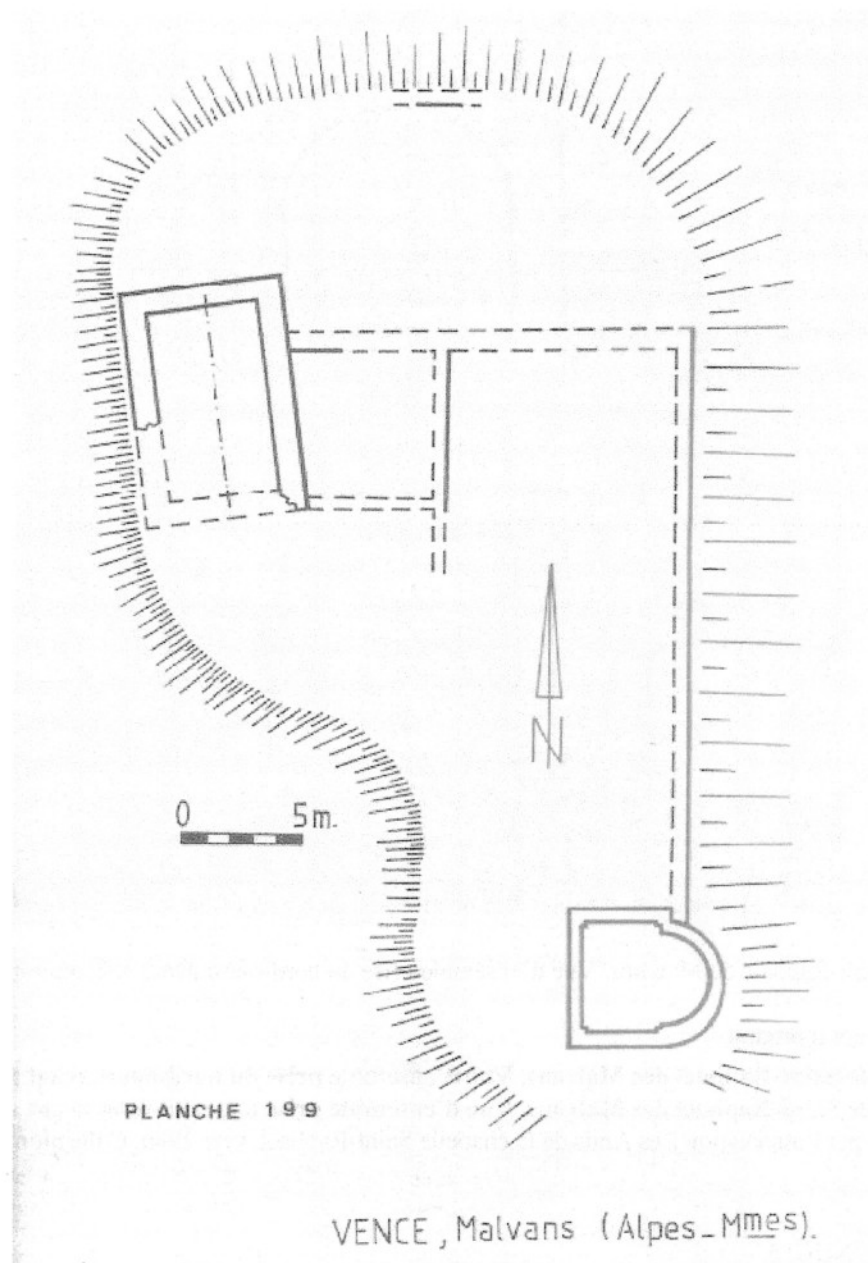
Planche n°199 : VENCE, Malvans (Alpes-Mmes). [Plan de l'enceinte avec le château et la chapelle].
